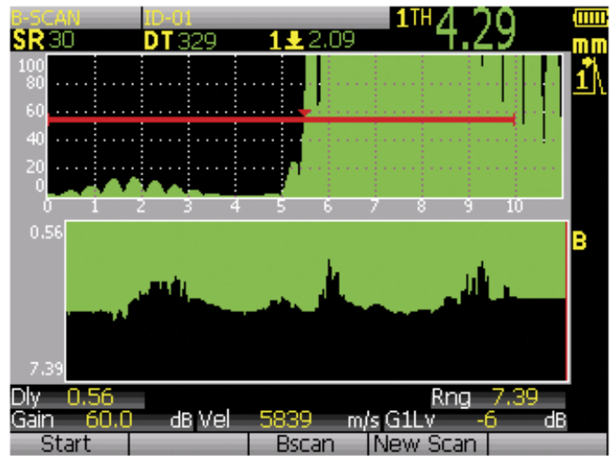
В-скан и плавающий строб
